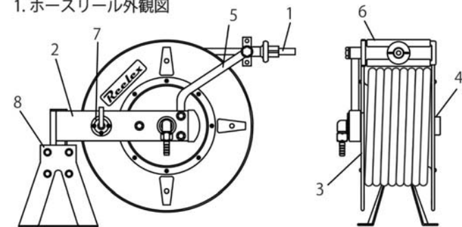
1. ホースリール外観図
