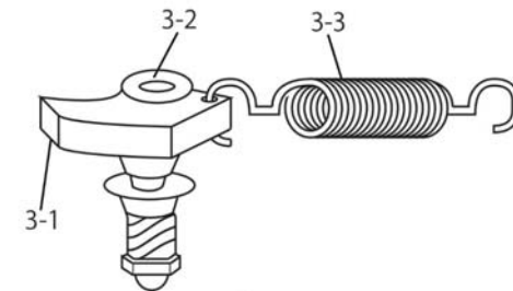
3. ラチェット Assy 拡大図
