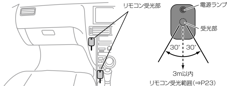
取付け例
